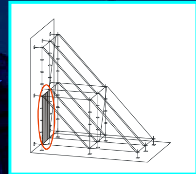
Schutzwände aus Bodenbelägen
