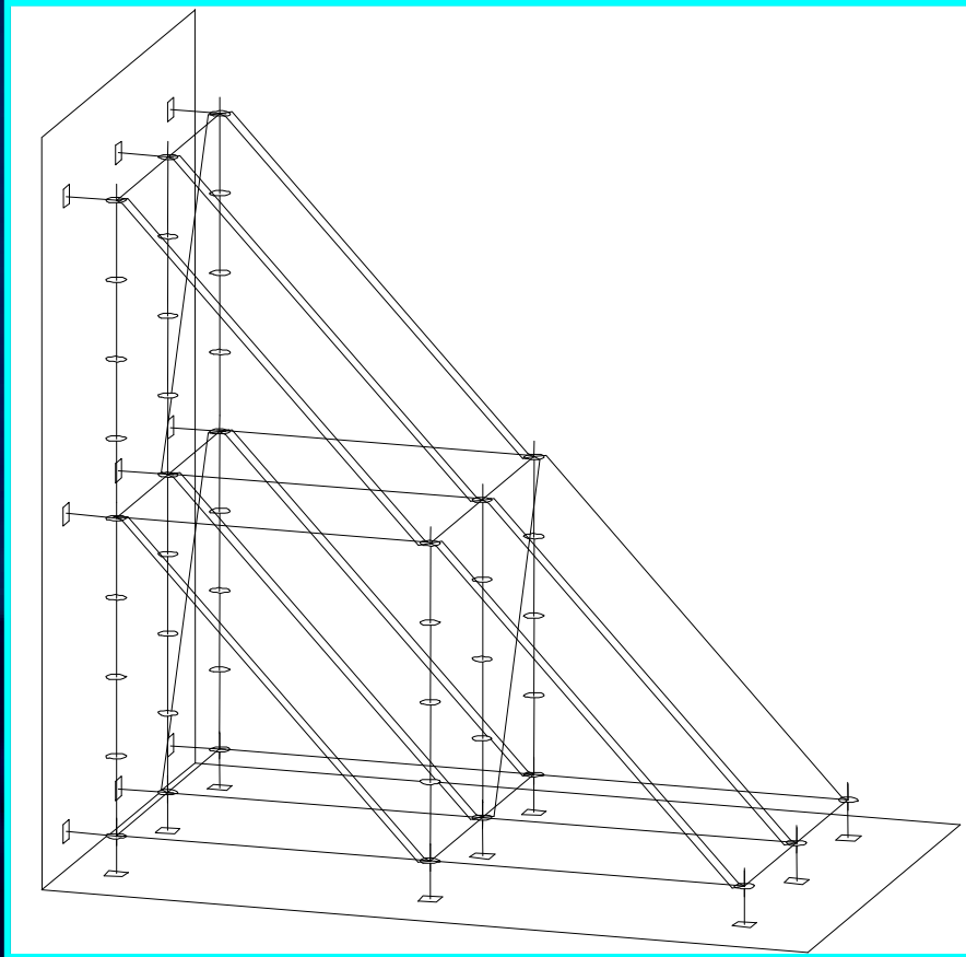
Strebstütze
