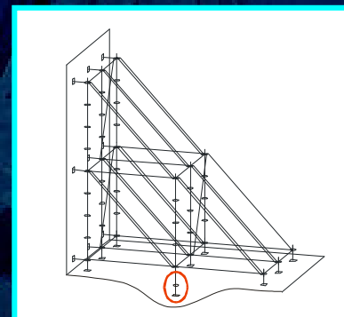
Auch auf unebenem/schrägen Grund
